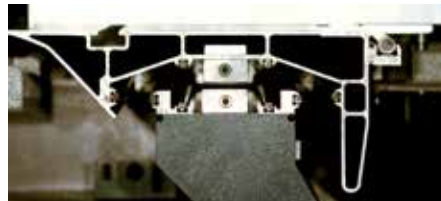
Zum Patent angemeldetes Schiebeschlittensystem
